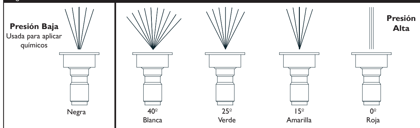
Figura 73 — Rocíe los Modelos del Rocío de Punta
