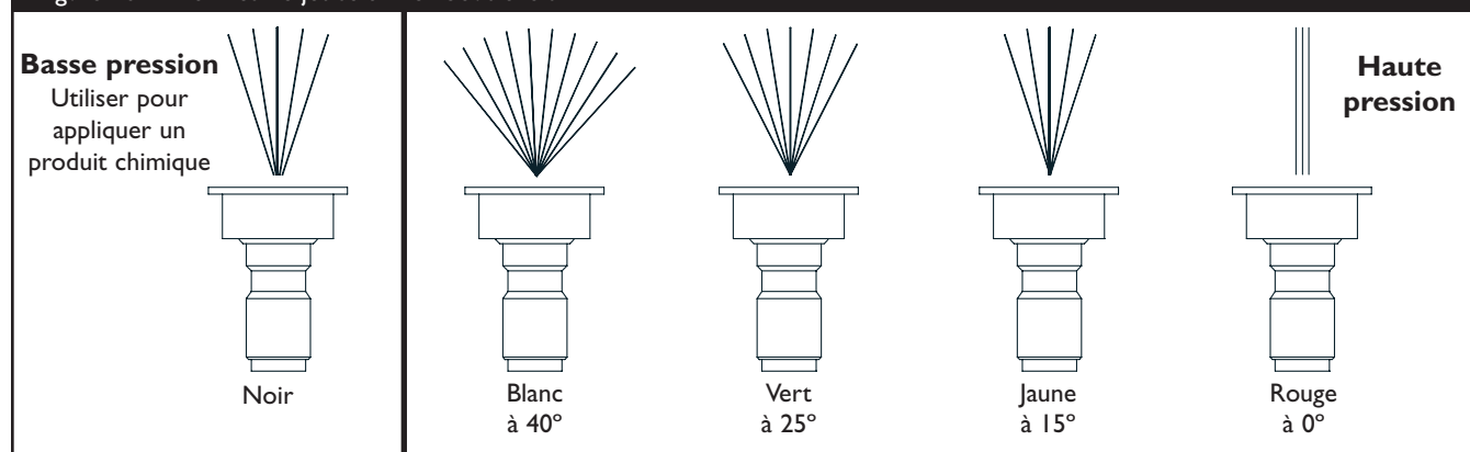
Figure 28 — Formes de jet selon l'embout choisi
