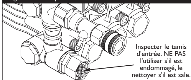
Figure 22 — Inspecter le tamis d'entrée
