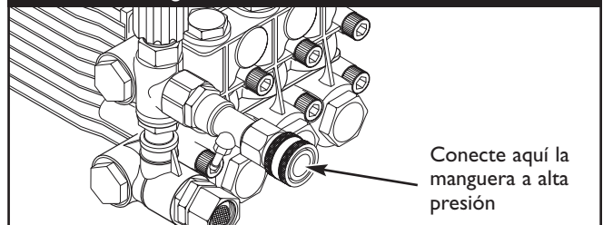
Figura 66 - Conectar la Manguera de Alta Presión a la Toma de Agua
