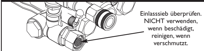
Abb. 37 - Einlasssieb überprüfen
