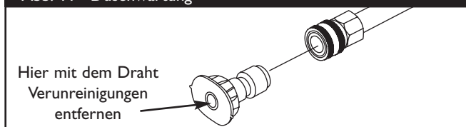
Abb. 44 - Düsenwartung
