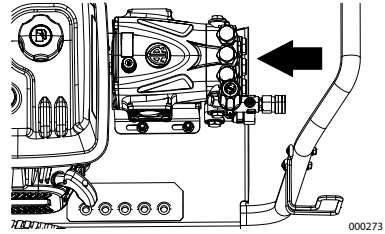
Figura 4-7. Empuje de la bomba hacia el motor
