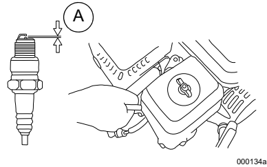
Figure 4-14. Bougie d'allumage
