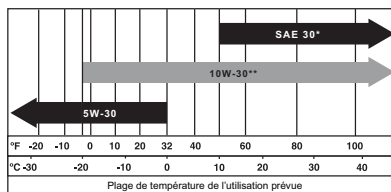
Figure 4-4. Viscosité d'huile
